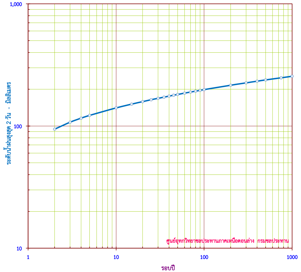
กราฟแสดง ปริมาณน้ำฝนสูงสุด 2 วัน ขนาดรอบปีต่างๆ สถานี 630181 อ.แม่สอด จ.ตาก
